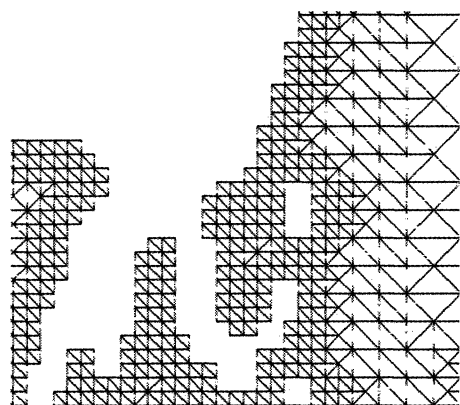
Рис. 1. Фрагмент триангуляции
