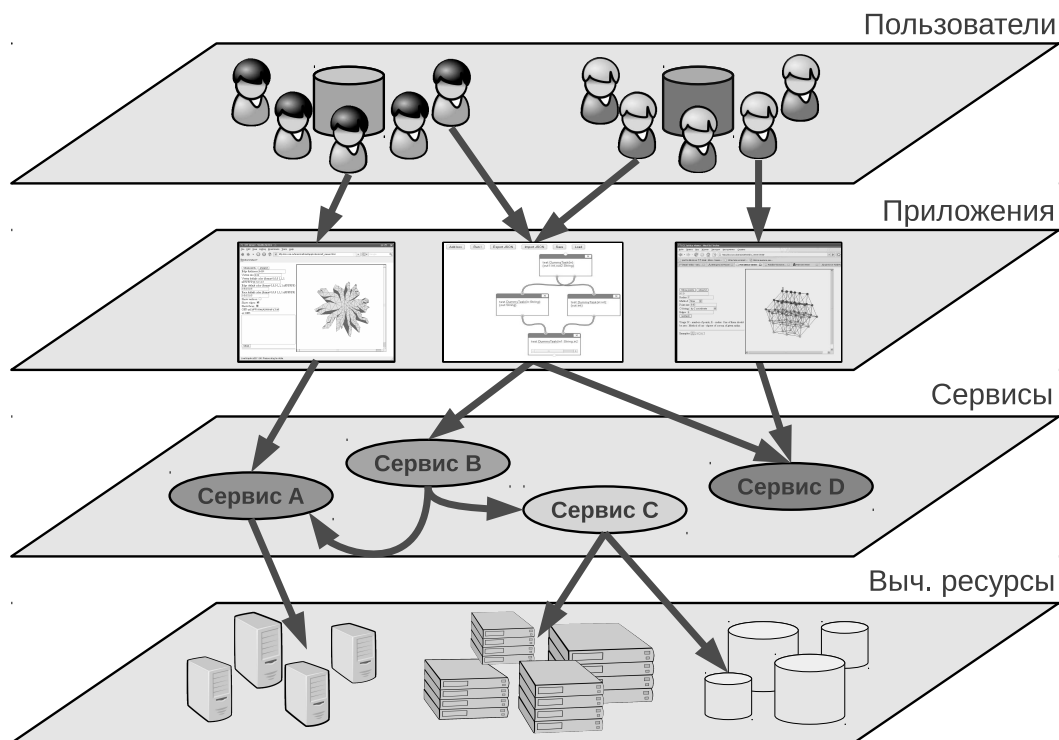
Рис. 1. Архитектура среды MathCloud
