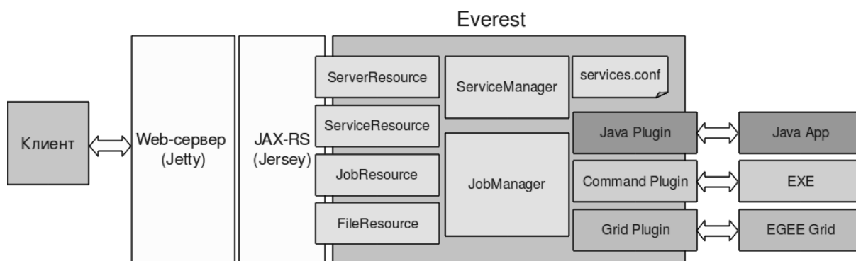
Рис. 2. Архитектура Everest
