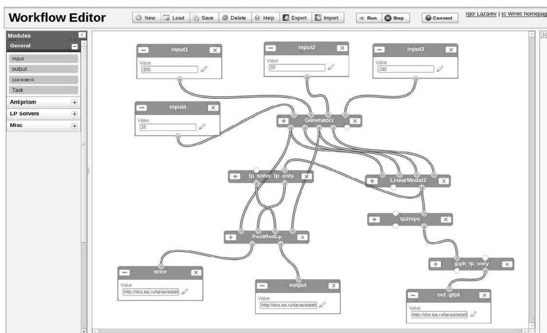
Рис. 3. Общий вид редактора сценариев
